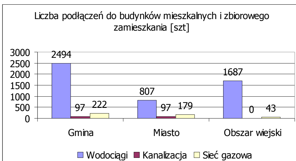
Wykres 16 Liczba połączeń prowadzących do budynków mieszkalnych i zbiorowego zamieszkania
