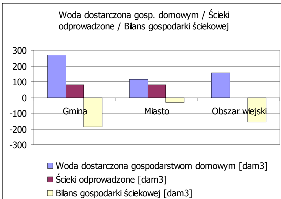
Wykres 17 Woda dostarczona gospodarstwu domowemu / Ścieki odprowadzone / Bilans gospodarki ściekowej
